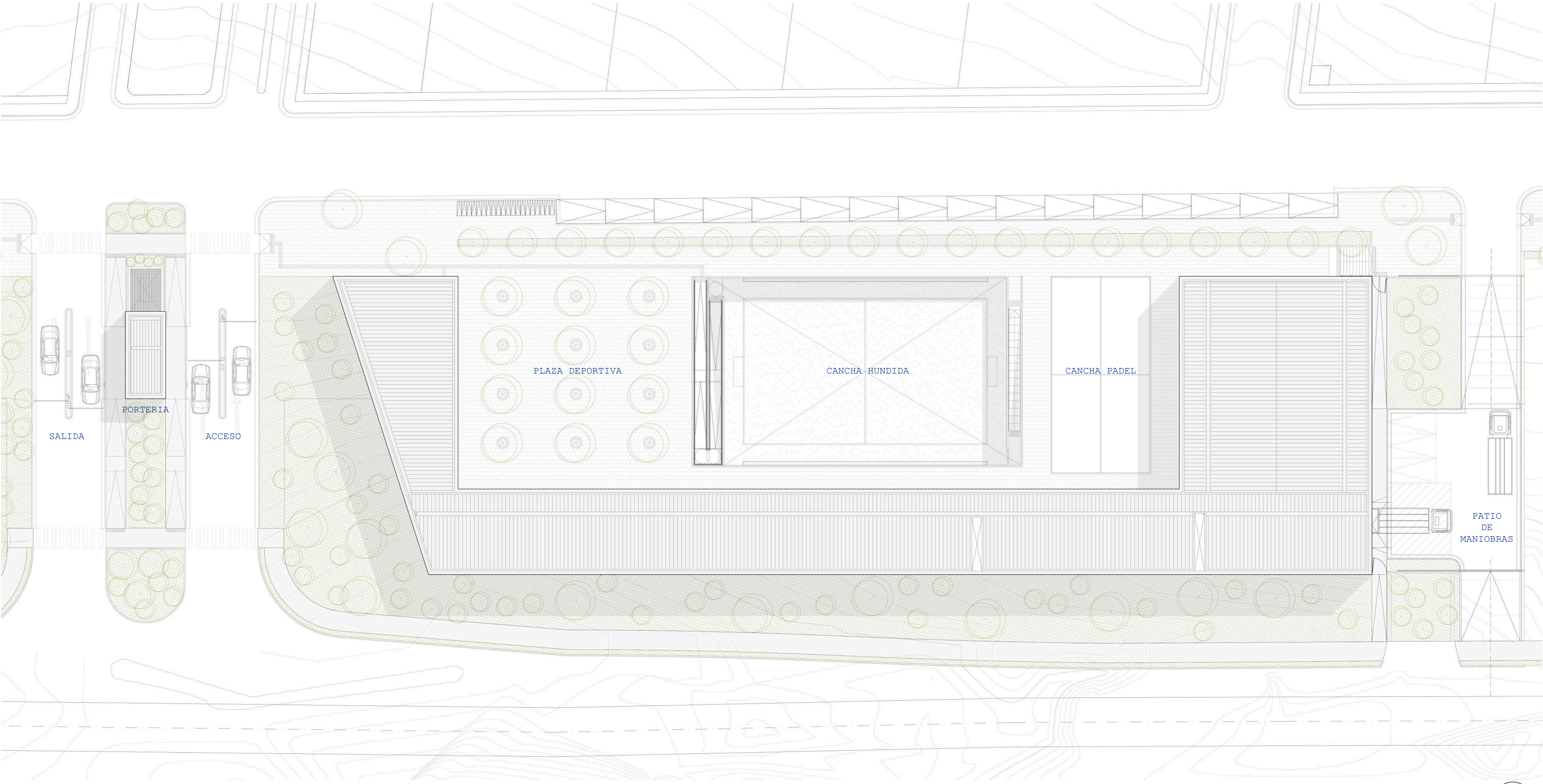
ADMINISTRACION PLANTA CUBIERTA
